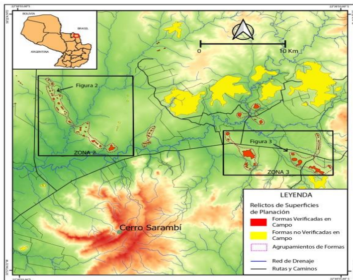
FIGURA 3: Mapa hipsométrico de la Zona 2 y 3, camino a Bella Vista Norte (Zona 2) y a la ciudad de Pedro Juan Caballero (Zona 3).E, donde se observan las geoformas más notables,
