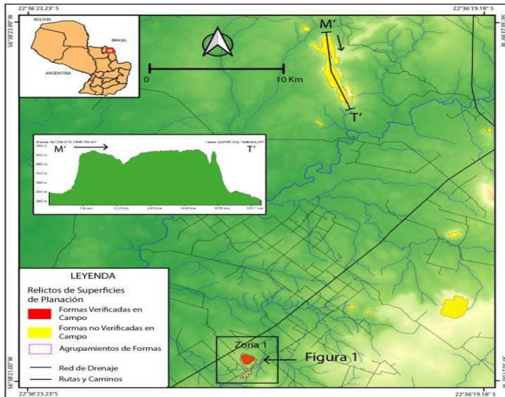
FIGURA 2: Mapa hipsométrico de la Zona 1. Se observa la localización del Cerro Memby (en rojo), que se interpreta como un relicto de una superficie de planación. Estas formas están agrupadas con otras más pequeñas dispuestas en dirección N-S (perfil topográfico M-T.)
