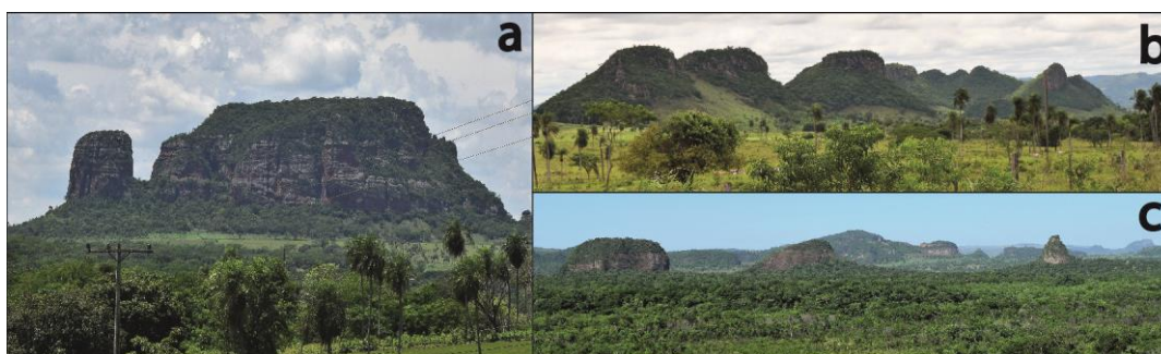
FIGURA 1: Relictos de una antigua paleosuperficie. (a) Vista del “Cerro Memby” en dirección E (Zona 1). (b) Vista panorámica en dirección E, desde la Ruta Nacional Número 3 correspondiente a la Zona 2, camino a Bella Vista Norte. (c) Vista panorámica en dirección SO desde el Cerro
